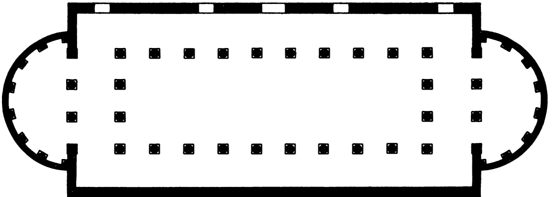
ichnographia basilicae Augustae Rauracorum prope Basileam sitae
